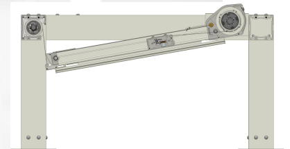
Croquis montage
